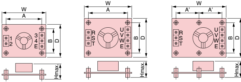
외형도1(단상입력)
