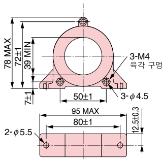
형식 F6045GB
