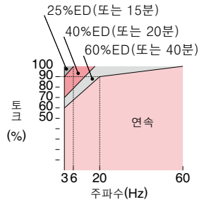
당사 표준모터의 허용부하 특성
