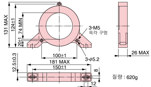
형식 F11080GB
