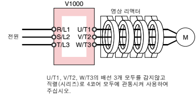
접속도 b
