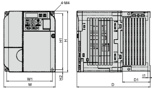
외형도 4
