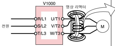
접속도 a
