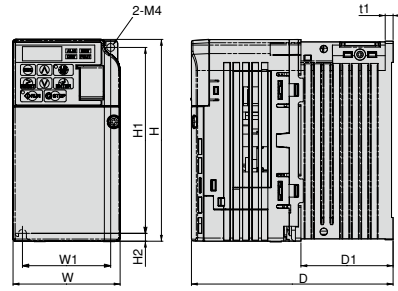
외형도 2
