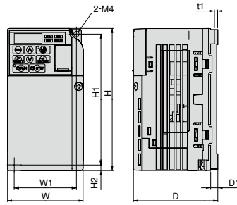
외형도 1
